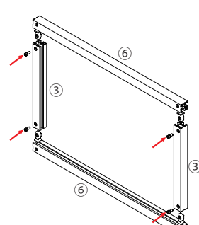
図 4-7 ↓ テーパードボルト(TB25)の向き
