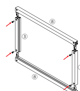
図 4-9 ↓ テーパードボルト(TB25)の向き
