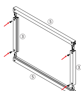
図 4-6 ↓ テーパードボルト(TB25)の向き
