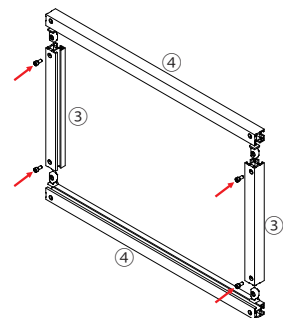
図 4-5 ↓ テーパードボルト(TB25)の向き
