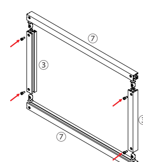
図 4-8 ↓ テーパードボルト(TB25)の向き
